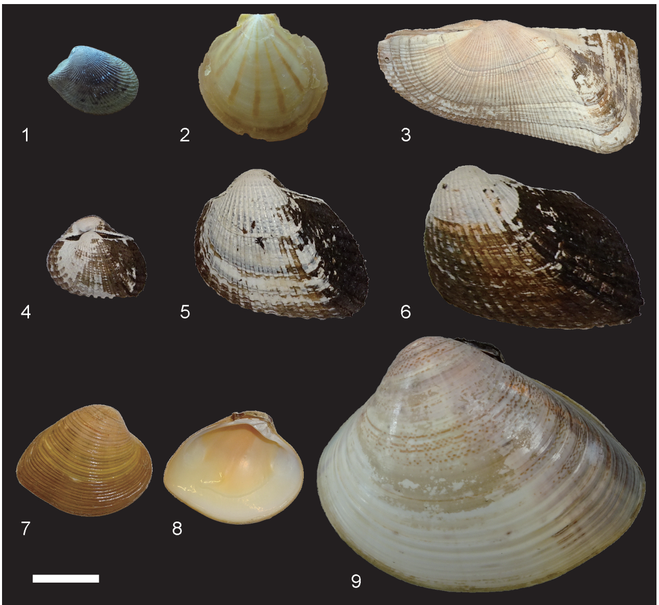
図2 展示用として収集した, 天草諸島および周辺海域より採集された二枚貝類の写真.
