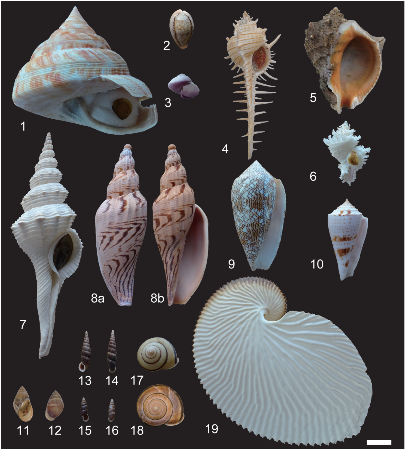
図1 展示用として収集した，天草諸島および周辺海域より採集された腹足類および頭足類の写真．
